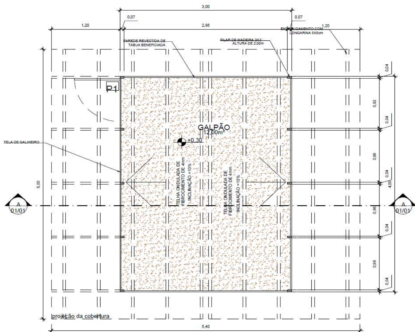
PLANTA BAIXA- AVIÁRIO A=12,00m 2 ESC. 1/50
